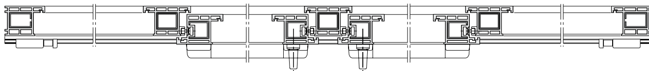
Festverglasung
